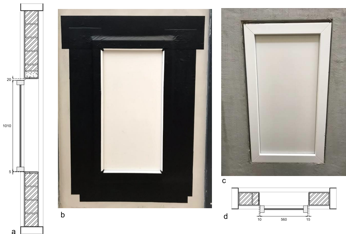
Figure 1: Montage d'essai, a. section transversale, b. face extérieure du mur, c. face intérieure du mur, d. section horizontale
